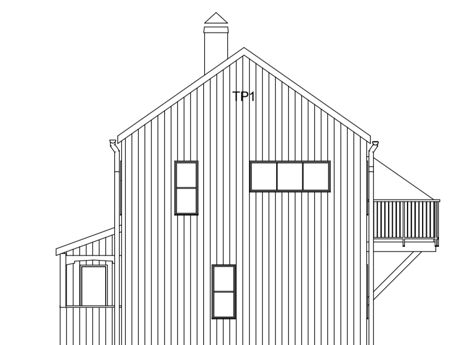
FASAD 4
