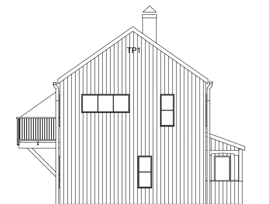
FASAD 2
